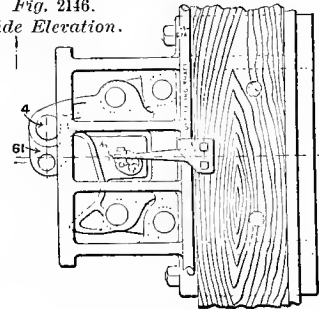
Fig. 2149. Plan.
